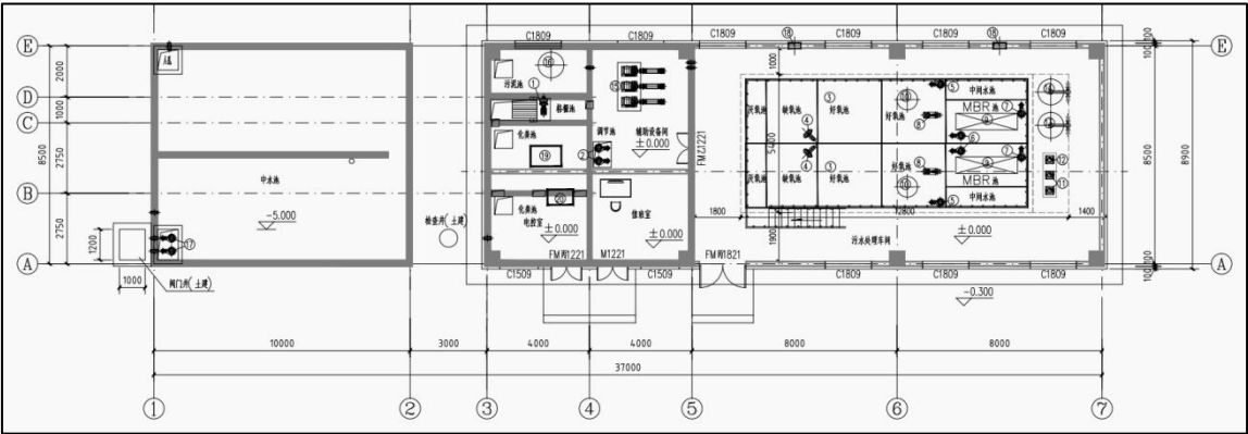
图6.3-1 污水处理设备平面布置图
