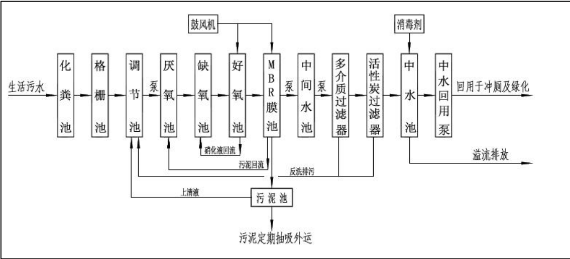
图6.3-2 污水处理工艺流程图
