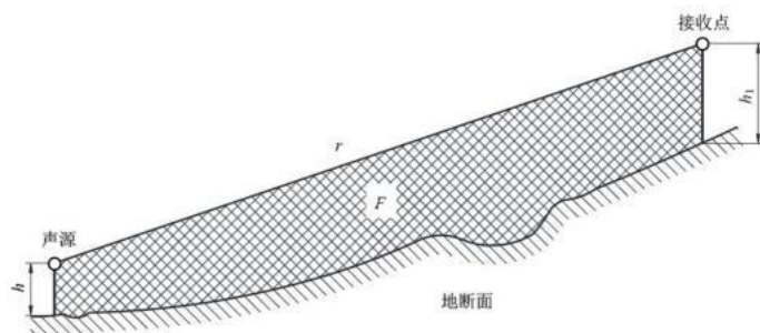
图 5.2-7 估计平均高度 h_m 的方法
